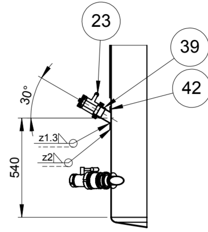
D-D SCALA (1 : 20)
